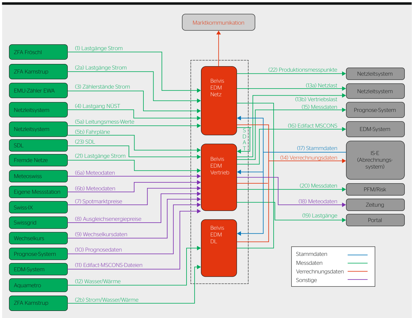
Bild 4 Übersicht über das System- und Schnittstellenkonzept.
